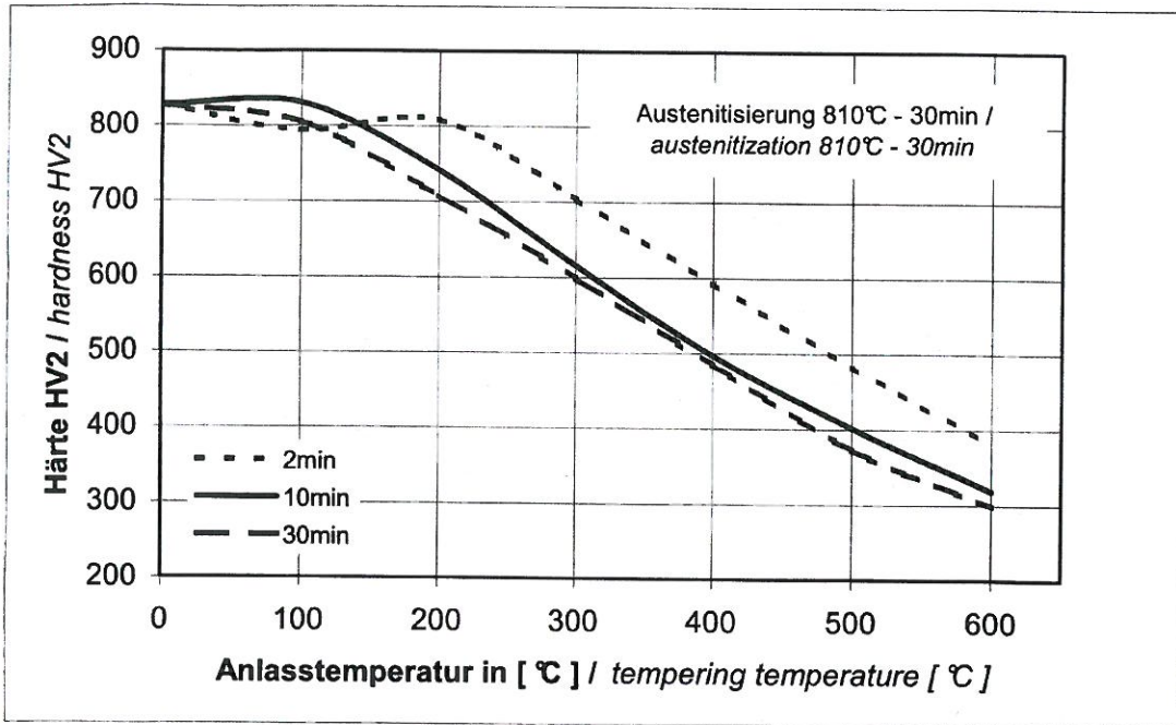
Anlasshärte des Stahles C75S (Variante 25) in Abhängigkeit von der Temperatur für unterschiedliche Haltezeiten
